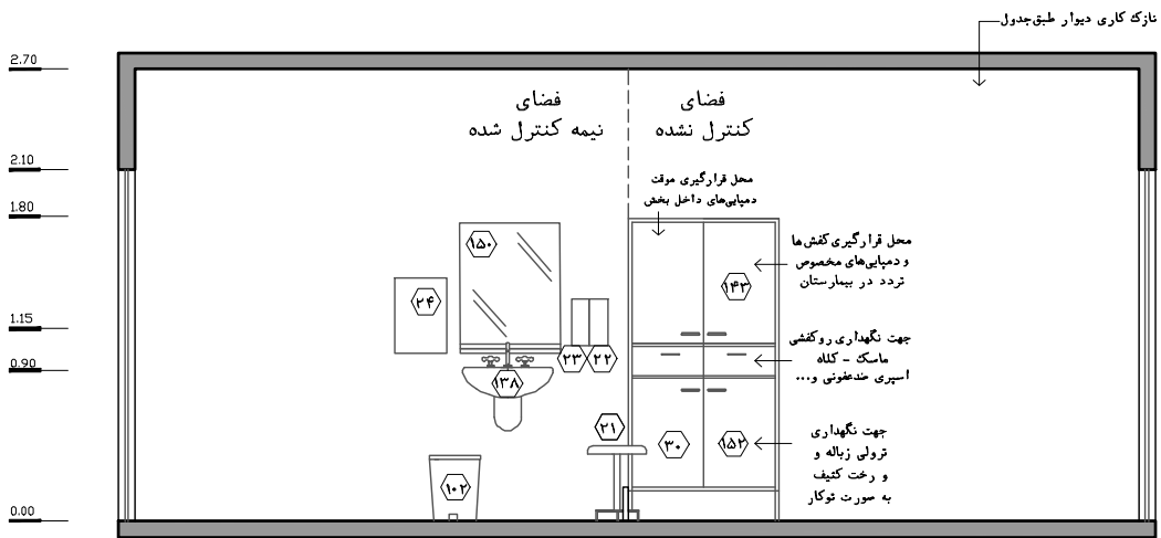
نقشه ۲-۱۵-۳- نمای ۳- مقیاس ۱:۵۰
