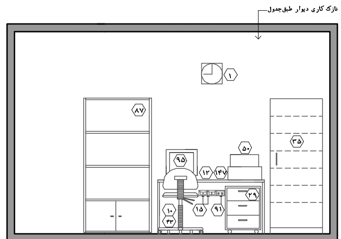
نقشه ۲-۷۶-۳- نمای ۳- مقیاس ۱:۵۰
