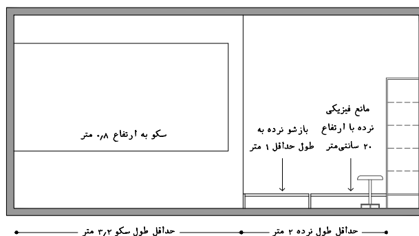
شکل ۲-۱۵- نمایشی از سکو در پیش‌ورودی بخش اعمال جراحی
