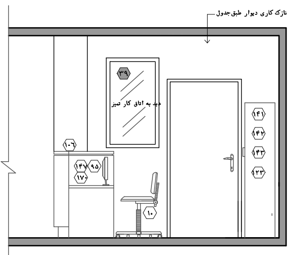
نقشه ۵۵-۲-۴- نمای ۴- مقیاس ۱:۵۰
