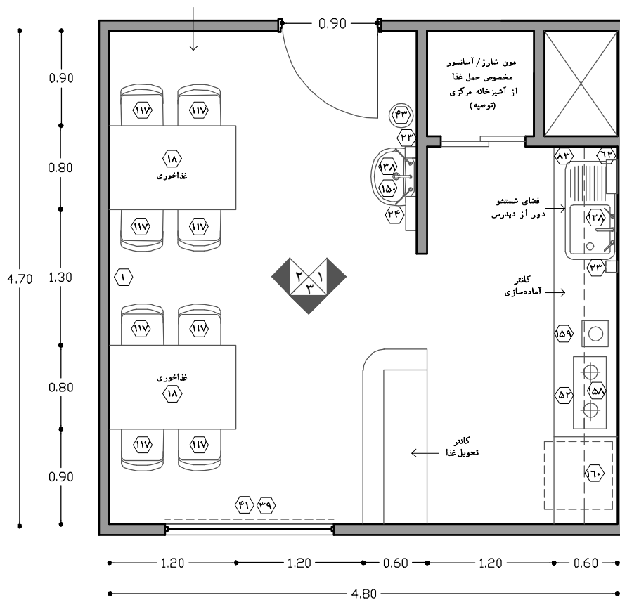
نقشه ۲-۱۲۲- پلان نمونه‌ی آبدارخانه در بخش‌های اعمال جراحی با ۹ اتاق عمل - مقیاس ۱:۵۰
