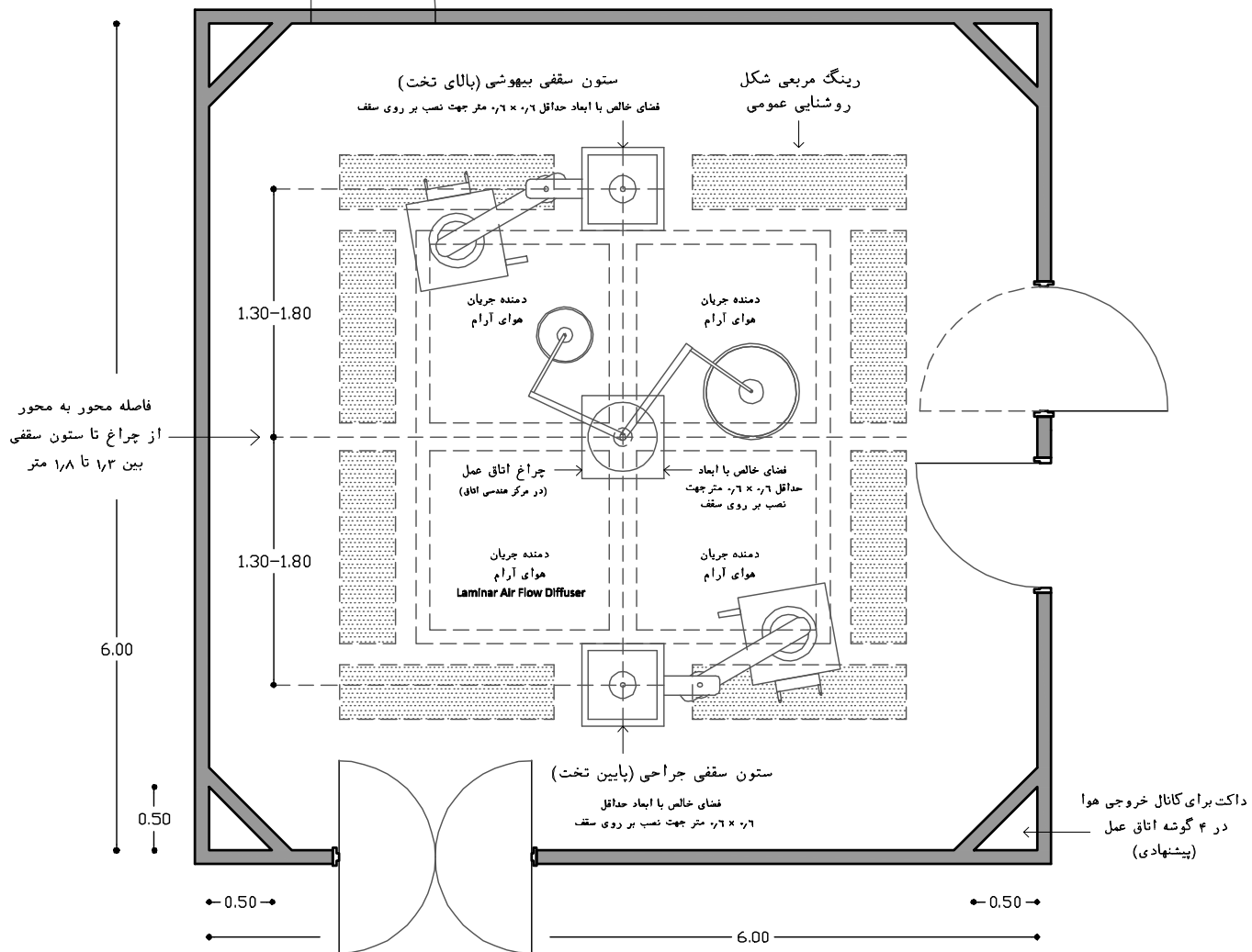
نقشه ۲-۱۵۰- پلان معکوس اتاق عمل جراحی کوچک - مقیاس ۱:۵۰
