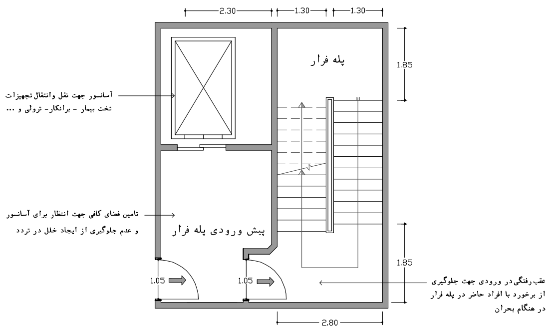
شکل ۲-۲۷- تعبیه آسانسور برانکاربر، در پیش‌ورودی پله‌های فرار
