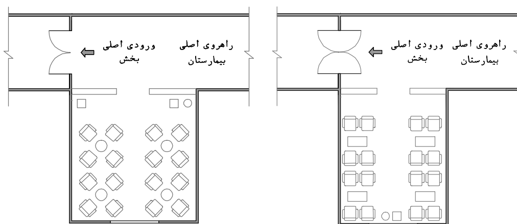
نقشه‌ی ۲-۴- چینش مبلمان به روش گروهی مقیاس ۱:۱۵۰
