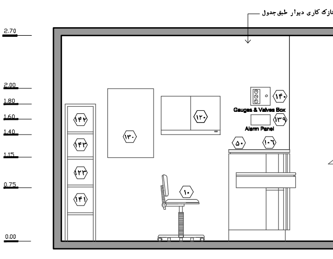
نقشه ۵۴-۲-۳- نمای ۳- مقیاس ۱:۵۰
