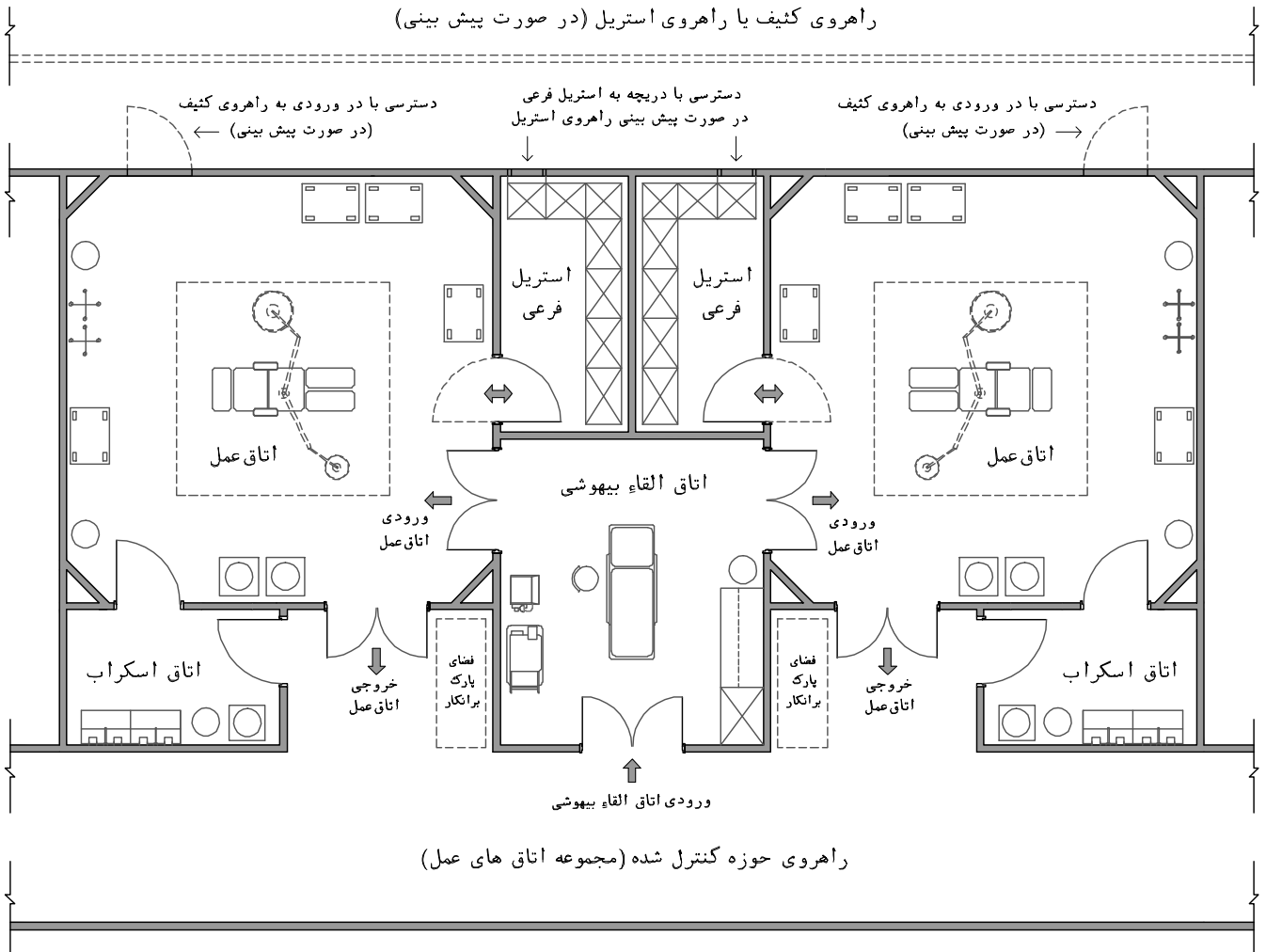
نقشه ۲-۱۳۷-پلان شماتیک اتاق القاء بیهوشی متصل به اتاق عمل از نوع مشترک- مقیاس ۱:۱۰۰
